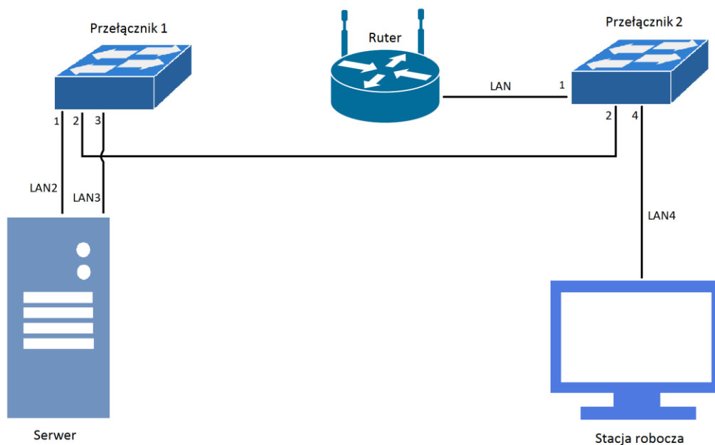
Schemat połączeń urządzeń w sieci lokalnej
